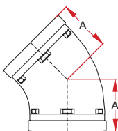
style 64 Coude 45°
